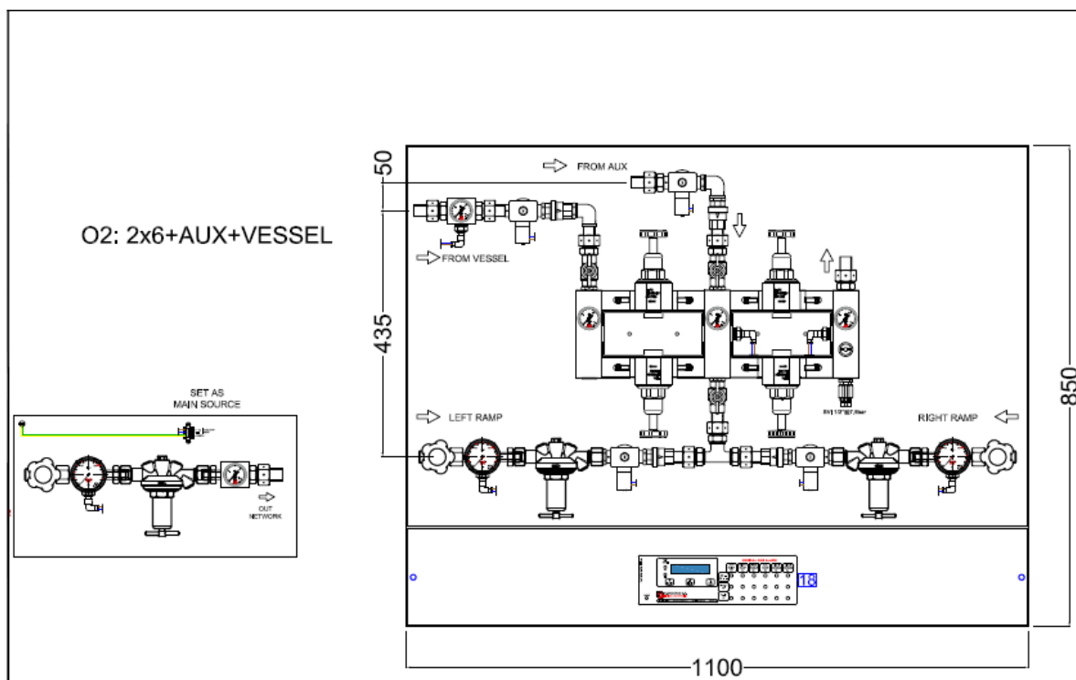
RYS 1 – Widok poglądowy nowoprojektowanego źródła tlenu
